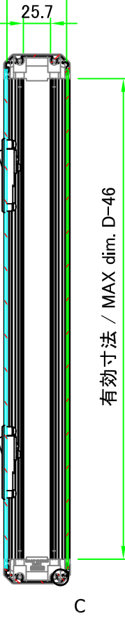
C: フレーム拡大図 / Frame cross-section
