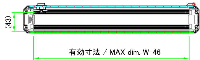
A-A (1:5)
